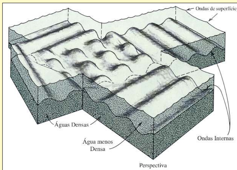
Figura 16: Ondas internas na interface entre duas camadas de água de densidades diferentes. Uma é densa (a mais baixa), a outra é menos densa (a superior). ( Oceanography [Oceanografia], Gross, p. 204.)
