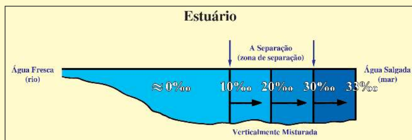
Figura 14: Seção longitudinal mostrando salinidade (partes por mil ‰) em um estuário. Podemos ver aqui essa divisória (zona de separação) entre a água fresca e a salgada. ( Introductory Oceanography [Oceanografia Introdutória], Thurman, p. 301, com um pequeno aperfeiçoamento.)
