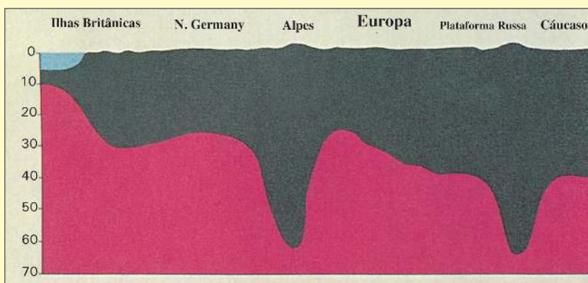
Figura 8: Seção esquemática. As montanhas, como as estacas, têm raízes profundas fincadas no solo. ( Anatomy of the Earth [Anatomia da Terra] , Cailleux, p. 220.)
