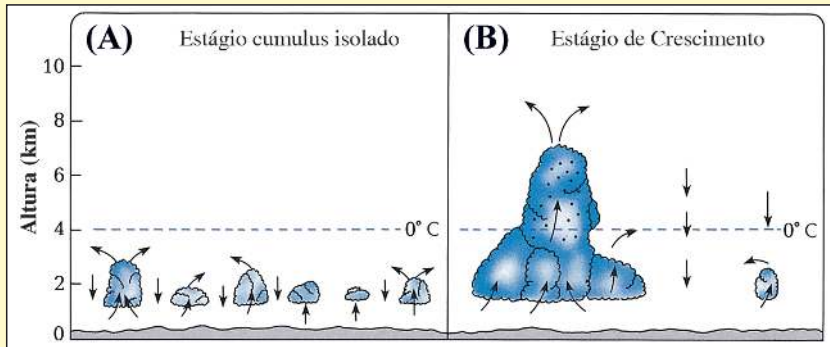
Figura 19: (A) Pequenos pedaços isolados de nuvens (nuvens cumulus). (B) Quando as pequenas nuvens se unem, as correntes de ar ascendentes dentro da nuvem maior aumentam, de modo que a nuvem é empilhada. Gotas de água são indicadas por · ( The Atmosphere [A Atmosfera], Anthes e outros, p. 269.)
