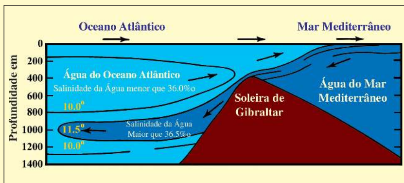
Figura 13: A água do mar Mediterrâneo quando entra no Atlântico pelo estreito de Gibraltar, com sua própria temperatura, salinidade e menor densidade características, por causa da barreira que as distingue. As temperaturas estão em graus Celsius (C°). ( Marine Geology [Geologia Marinha], Kuenen, p. 43, com um pequeno aperfeiçoamento.)
