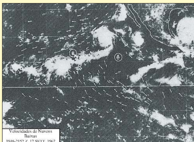
Figura 17: Foto de satélite mostrando as nuvens se movendo na direção das áreas de convergência B, C e D. As setas indicam as direções do vento. ( The Use of Satellite Pictures in Weather Analysis and Forecasting [O Uso de Fotos de Satélite na Análise e Previsão do Tempo], Anderson e outros, p. 188.)
