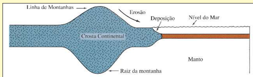
Figura 9: Outra ilustração mostra como as montanhas têm forma de estacas, devido às suas raízes profundas. ( Earth Science [Ciência da Terra] , Tarbuck e Lutgens, p. 158.)
