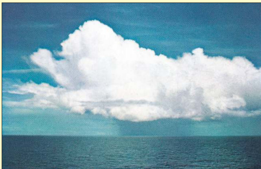
Figura 21: Uma nuvem cumulonimbus. ( A Colour Guide to Clouds [Um Guia Colorido para as Nuvens], Scorer e Wexler, p. 23.) Deus disse no Alcorão:
