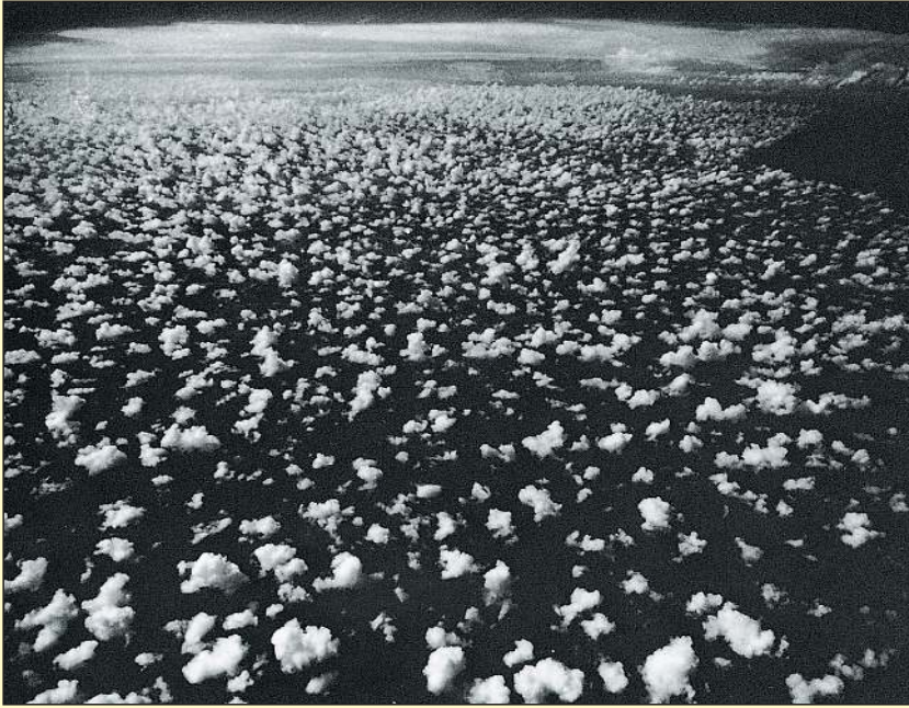
Figura 18: Pequenos pedaços de nuvens (nuvens cumulus) se movendo na direção de uma zona de convergência próxima ao horizonte, onde podemos ver uma grande nuvem cumulonimbus. ( Clouds and Storms [Nuvens e Tempestades], Ludlam, ilustração 7.4)
