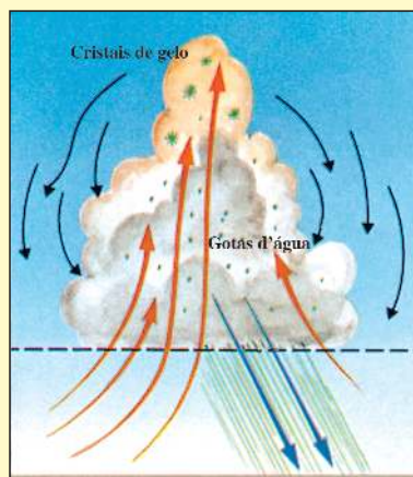
Figura 20: Uma nuvem cumulonimbus. Depois que a nuvem é empilhada, a chuva começa. ( Weather and Climate [Clima e Temperatura], Bodin, p. 123.)
