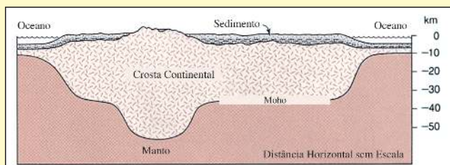
Figura 7: Montanhas têm raízes profundas sob a superfície do solo. ( Earth [Terra] , Press e Siever, p. 413.)
