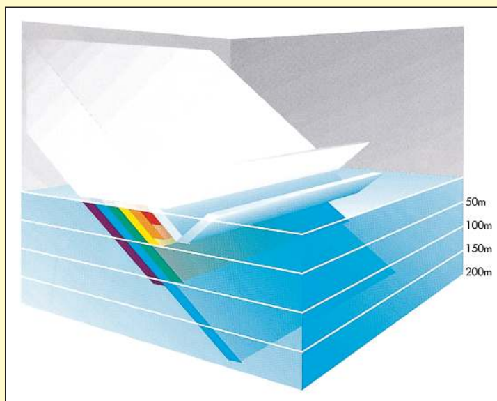
Figura 15: Entre 3 e 30 por cento da luz solar é refletida na superfície do mar. Então quase todas as sete cores do espectro de luz são absorvidas uma após a outra nos primeiros 200 metros, exceto a luz azul. ( Oceans [Oceanos], Elder e Pernetta, p. 27.)
